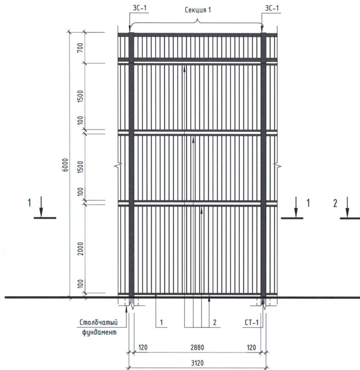
Схема ограждения спортивных площадок
