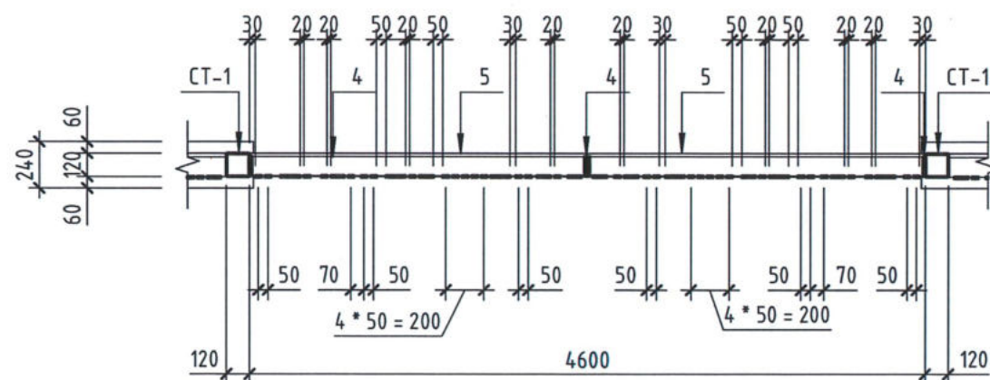
Сечение 3-3
