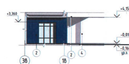
Фрагмент фасада 4
