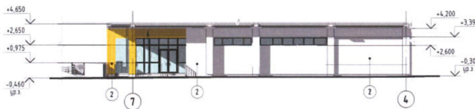
Фрагмент фасада 2
