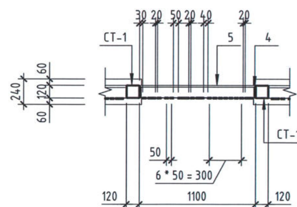
Сечение 2-2
