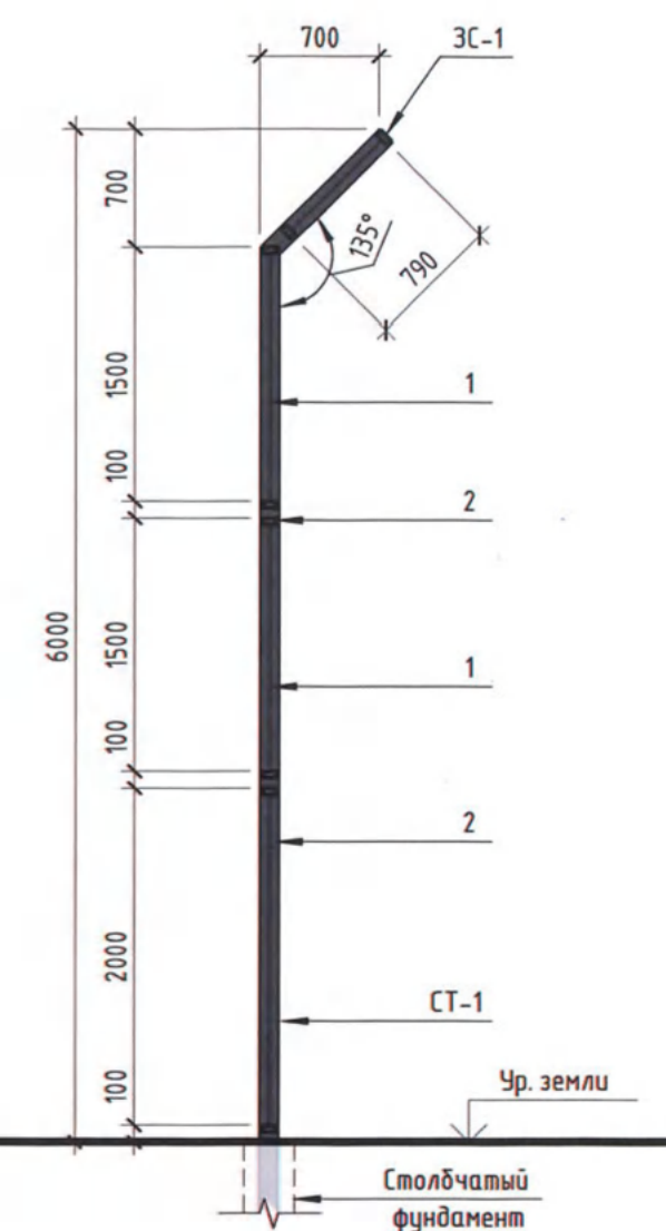
Сечение 3-3
