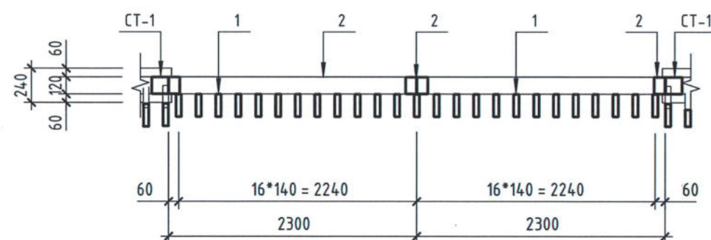
Сечение 2-2
