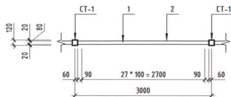
Сечение 1-1
