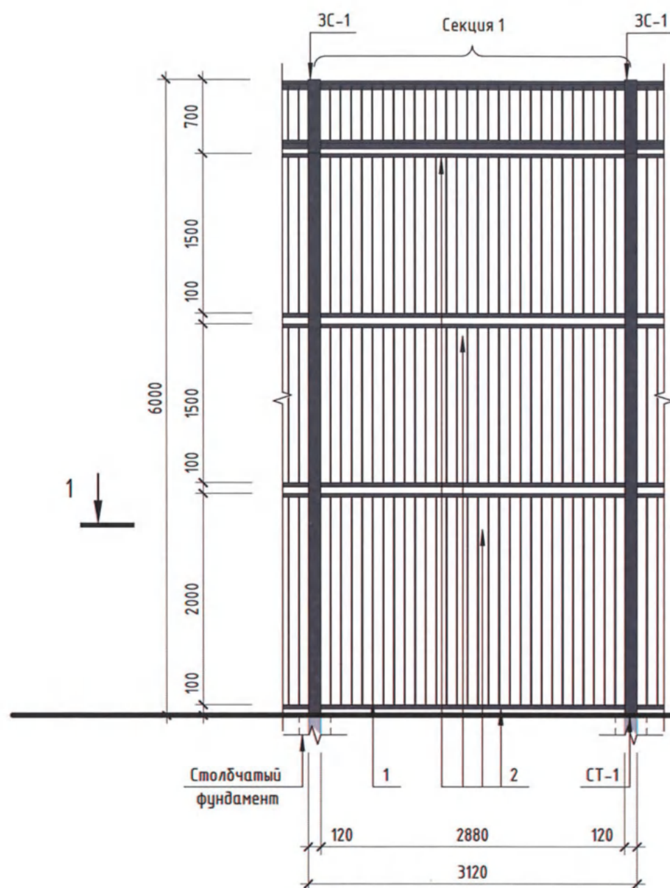
Схема ограждения спортивных площадок
