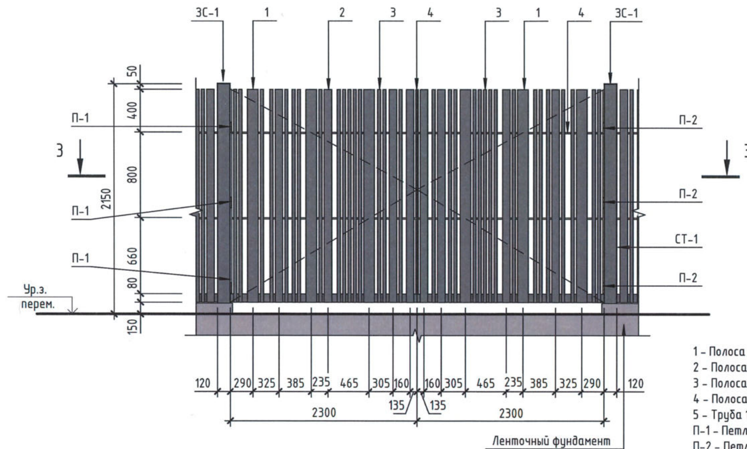
Схема распашных-автоматических ворот
