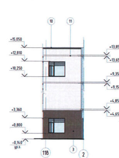
Фрагмент фасада 5
