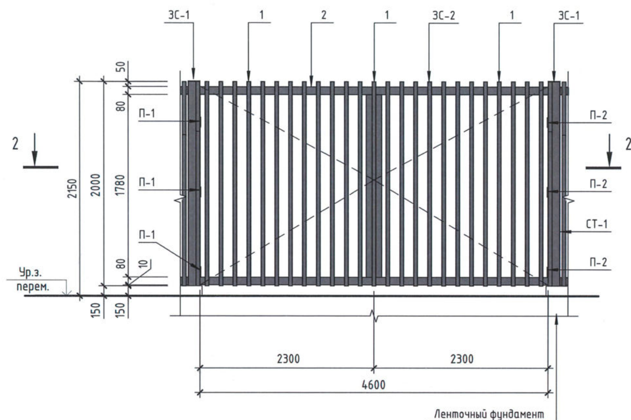
Схема распашных автоматических ворот
