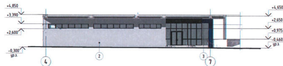
Фрагмент фасада 1
