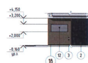
Фрагмент фасада 3
