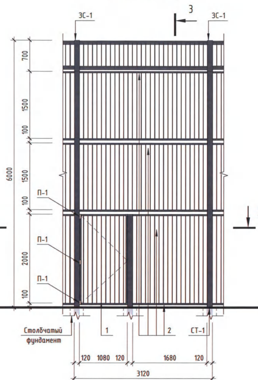
Схема калитки
