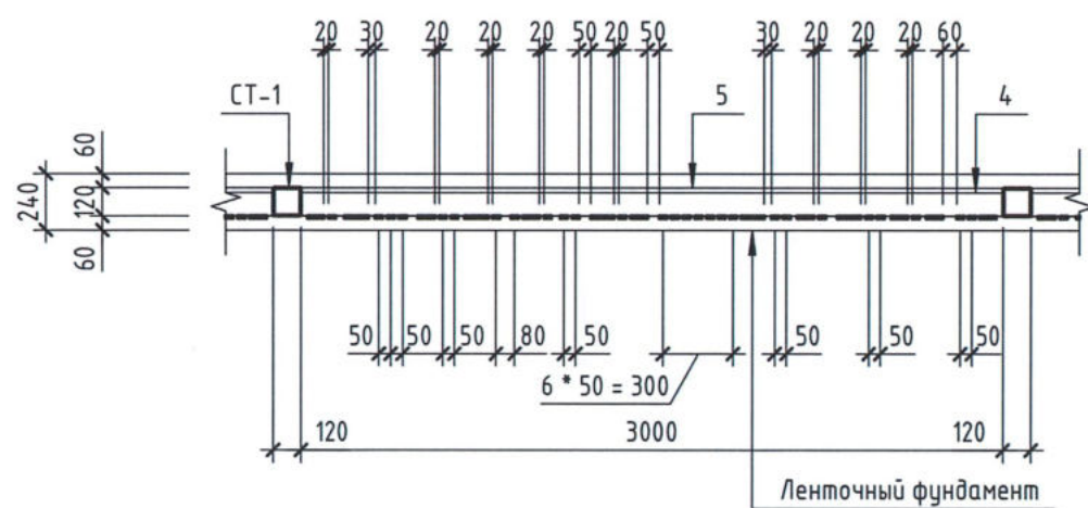
Сечение 1-1
