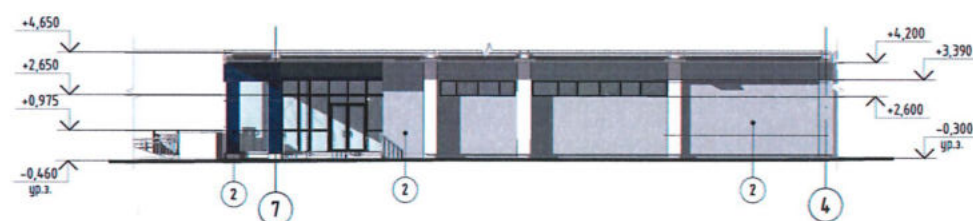
Фрагмент фасада 2
