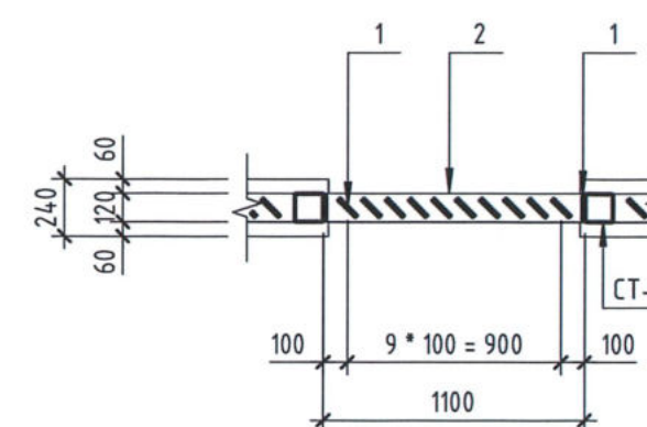
Сечение 2-2
