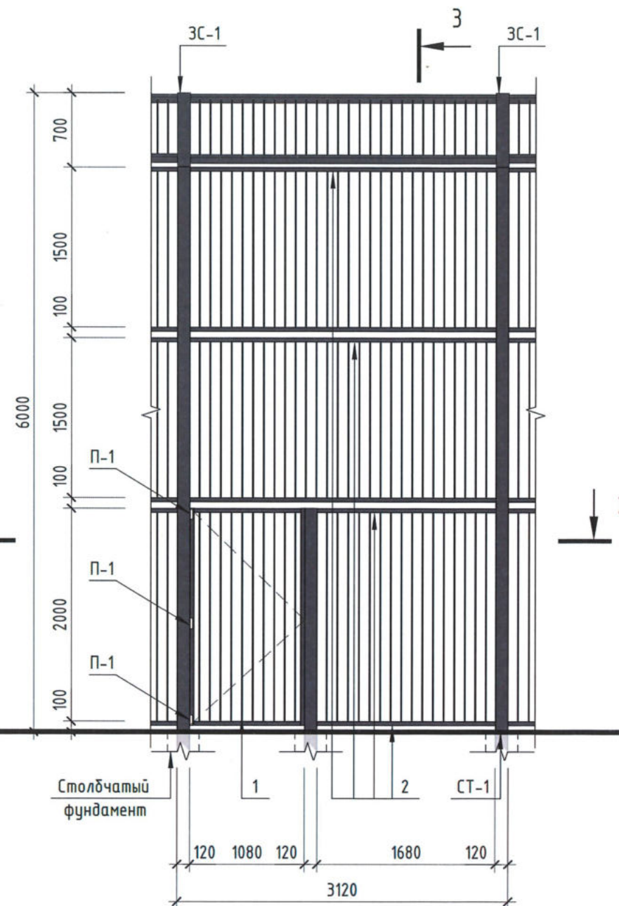
Схема калитки
