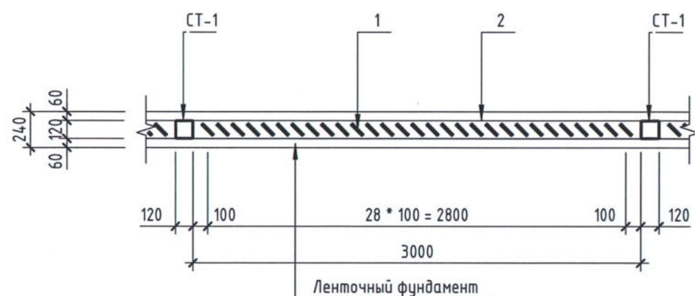
Сечение 1-1
