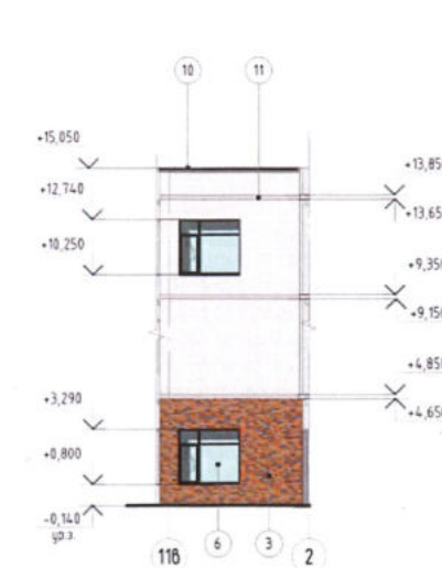
Фрагмент фасада 5
