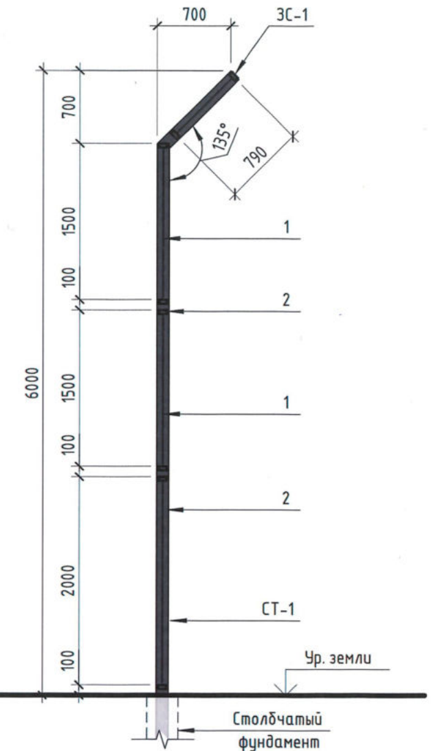
Сечение 3-3
